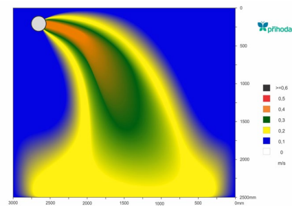
Patrones de flujo de aire, microperforación 90^\circ , 165 Pa
